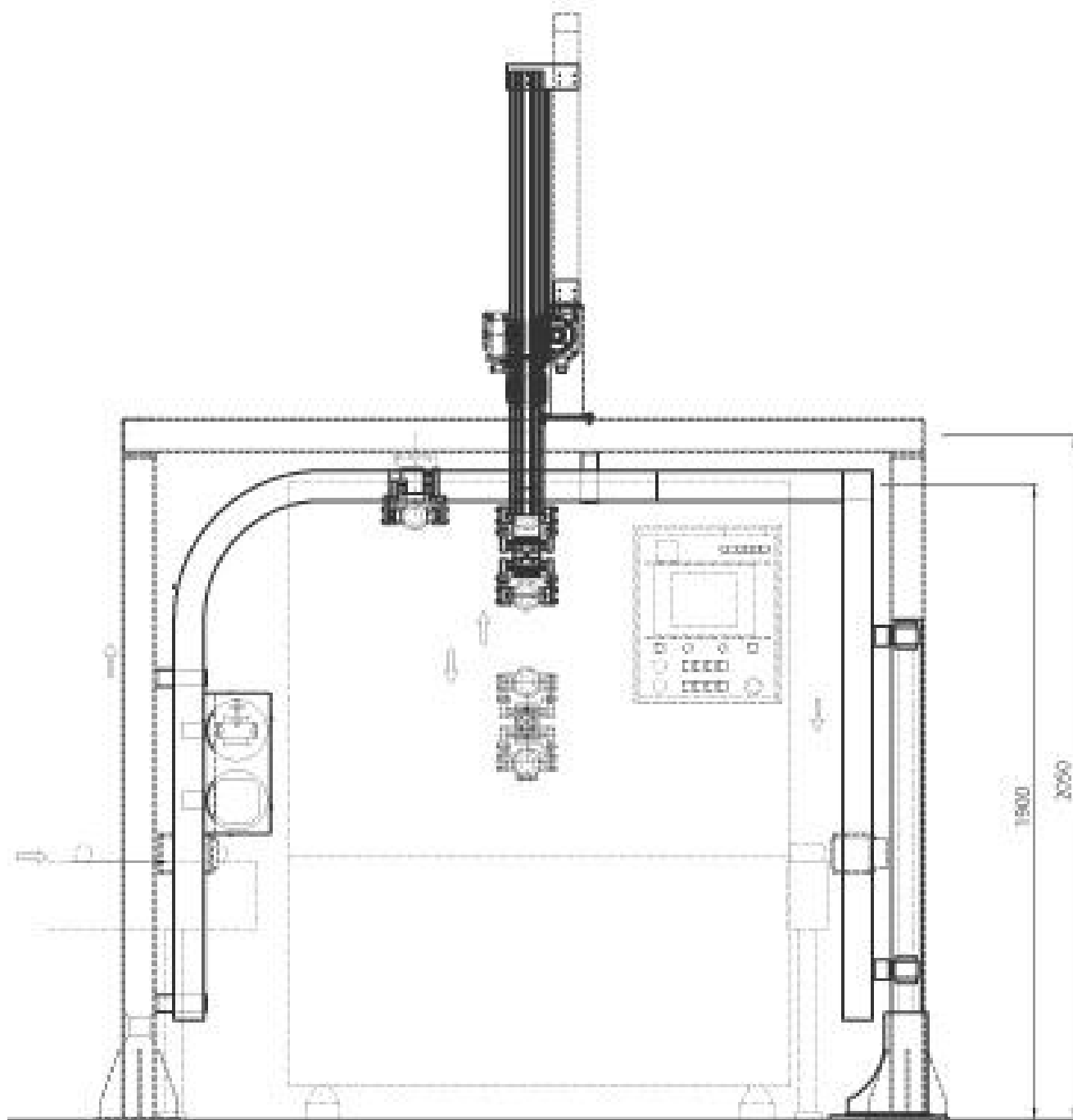
立面图 1
